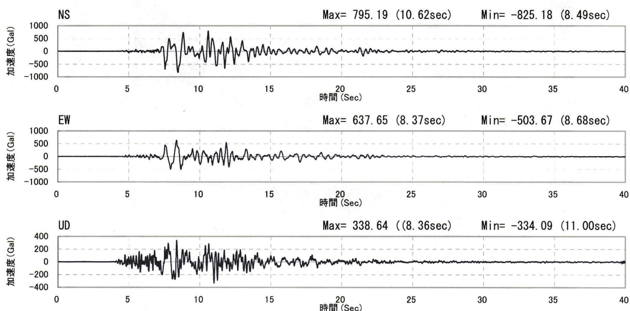
加速度波形
