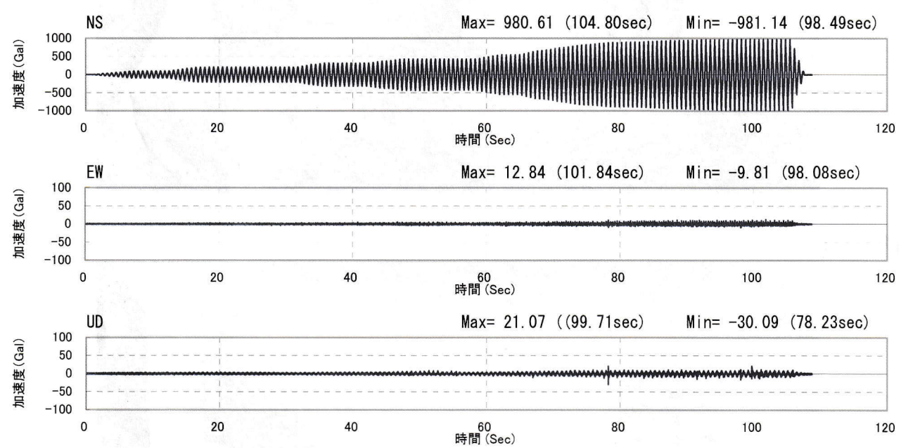
加速度波形
