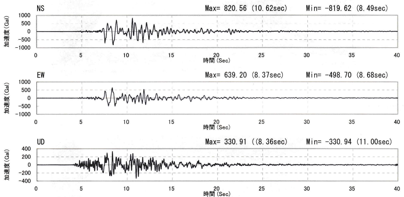
加速度波形
