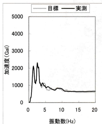
加速度応答スペクトル
